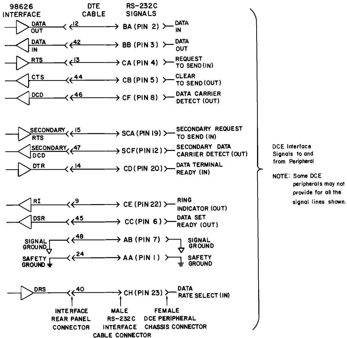
DTE Cable Diagram
